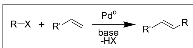
Figura 29: La reazione di Heck
