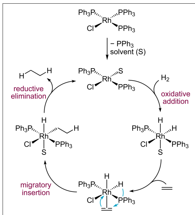
Figura 28: Step del funzionamento del catalizzatore di Wilkinson
