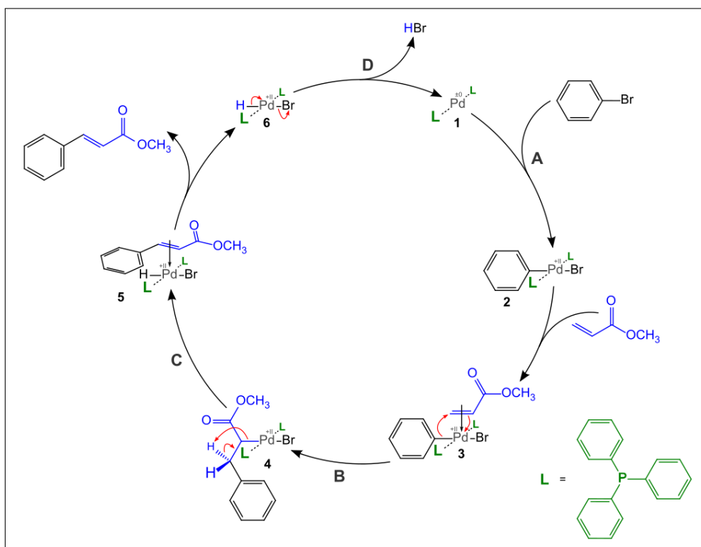
Figura 30: Step del funzionamento del catalizzatore di Heck
