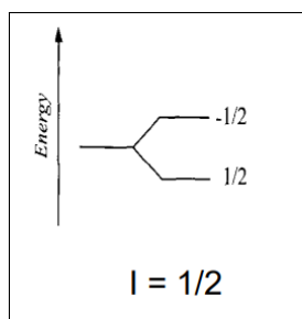
Figura 38: Stati possibili per un nucleo di spin \frac{1}{2} : \frac{1}{2} = \alpha , -\frac{1}{2} = \beta
