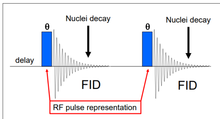
Figura 40: Rappresentazione di una Pulse Sequence in NMR
