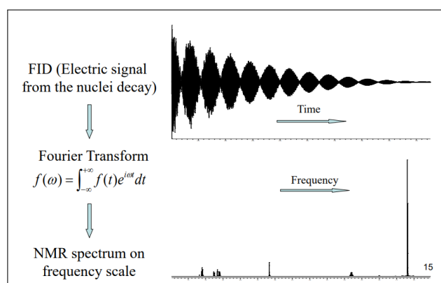
Figura 41: Algoritmo di gestione di uno FT-NMR
